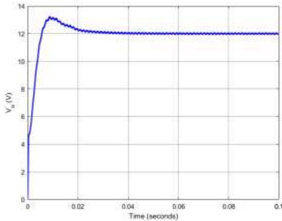
Fig. 7. Output voltage
