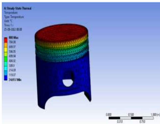
Fig 8.2.2 (d) Al Alloy under Temperature
