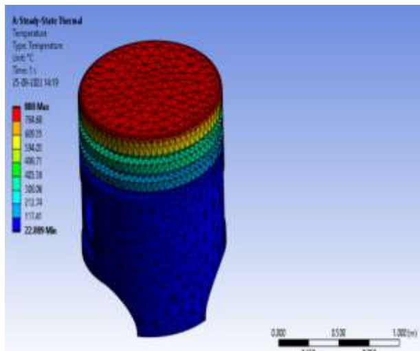
Fig 8.2.1 (d) Cast Iron under Temperature
