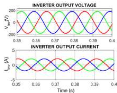
Fig. 15. Inverter output
