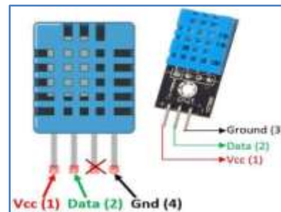
Fig. 3. DHT11SensorModule
