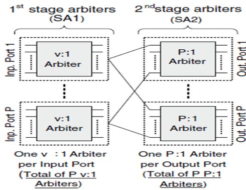
Fig. 6. Switch Allocation (SA) Unit.
