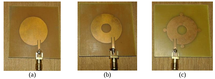
Fig. 7. Fabricated geometry of (a) 0th iteration (b) Ist iteration (c) IInd iteration
