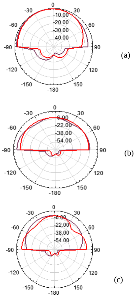
Fig. 5. Simulated radiation pattern of Ist iteration at (a) 3.10GHz (b) 7.76 GHz
