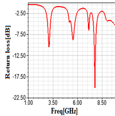
(b) Ist iteration stage,
