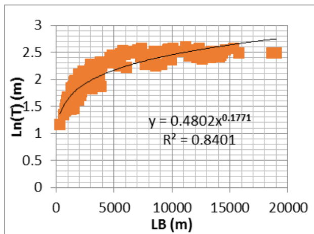
FIG. 27: LOGe(T) TO LxB REGRESSION.
