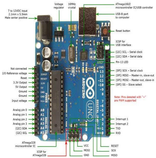
Figure 5- Arduino UNO
