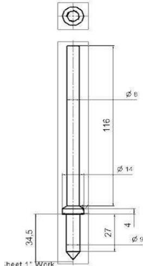
Fig. 6 Valve Rod
