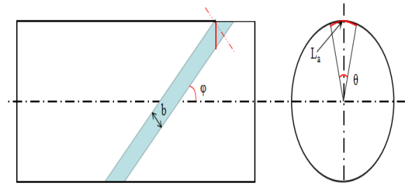
Fig.3 Filament winding parameter
