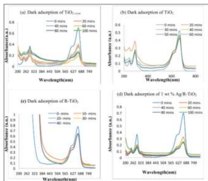
Fig. 7. Dark absorption of (a) \text{TiO}_{2\text{cryst}} (b) \text{TiO}_2 (c) \text{R-TiO}_2 and (d) 1 wt% \text{Ag/R-TiO}_2 .
