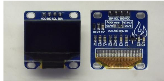
Fig 3:- OLED Display
