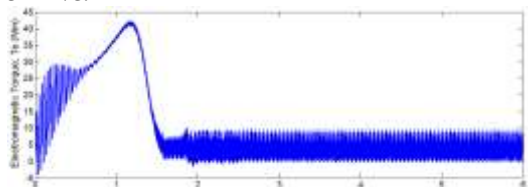
Fig. 25. Rotor Torque
