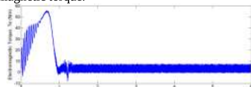
Fig. 22. Rotor Torque
