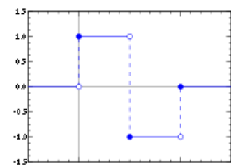
Fig 4: Haar wavelet
