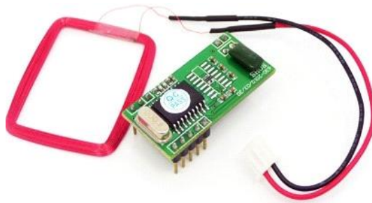
Fig 2 RFID Reader
