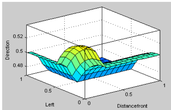
c-path 3
