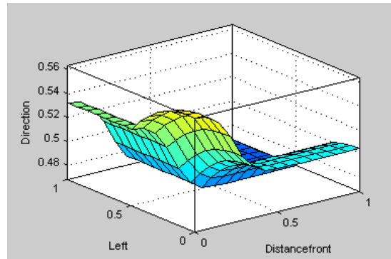
b- path 2
