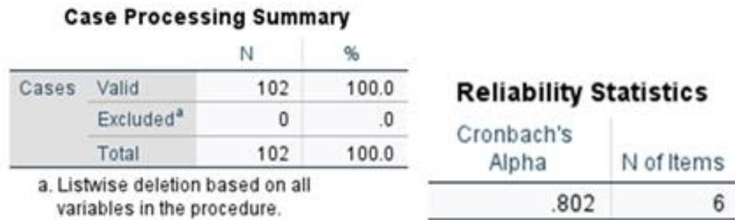
Fig. 16. Cronbach alpha (a) (RO2)
