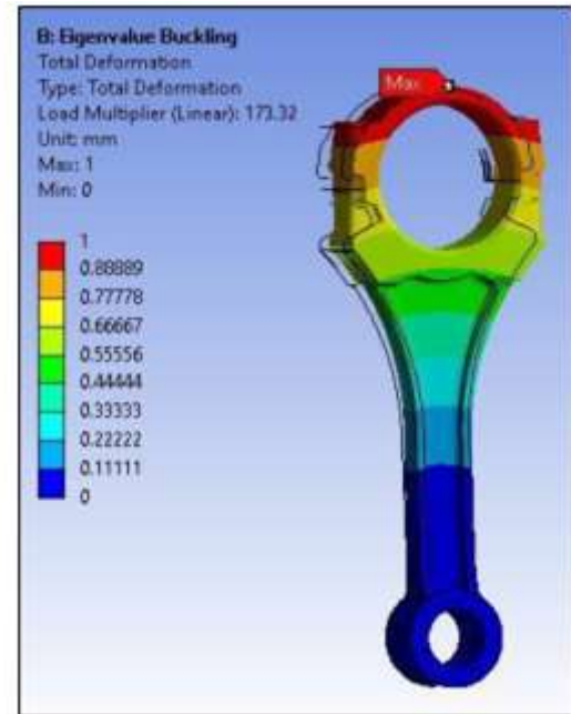
Fig. 13. Buckling Result
