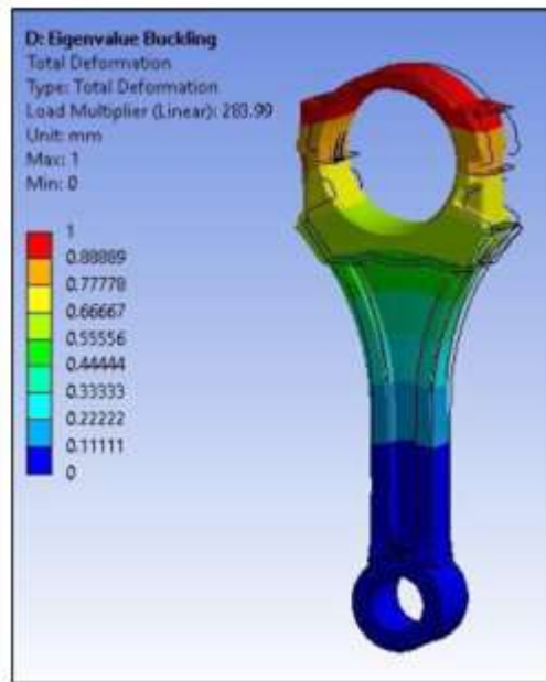
Fig. 18. Buckling Result
