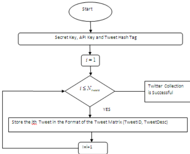
Fig. 5. Data Collection using Twitter
