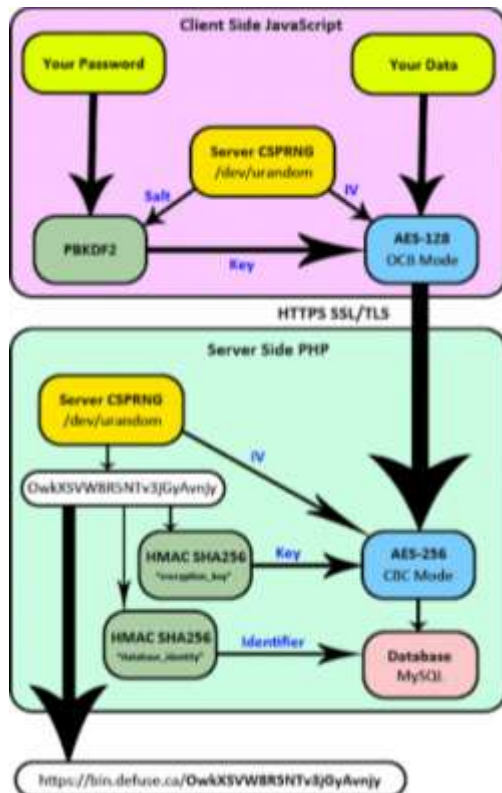
Fig 2.6 DFD
