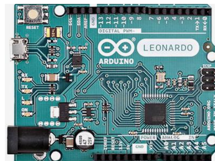
Fig1.Arduino Leonardo
