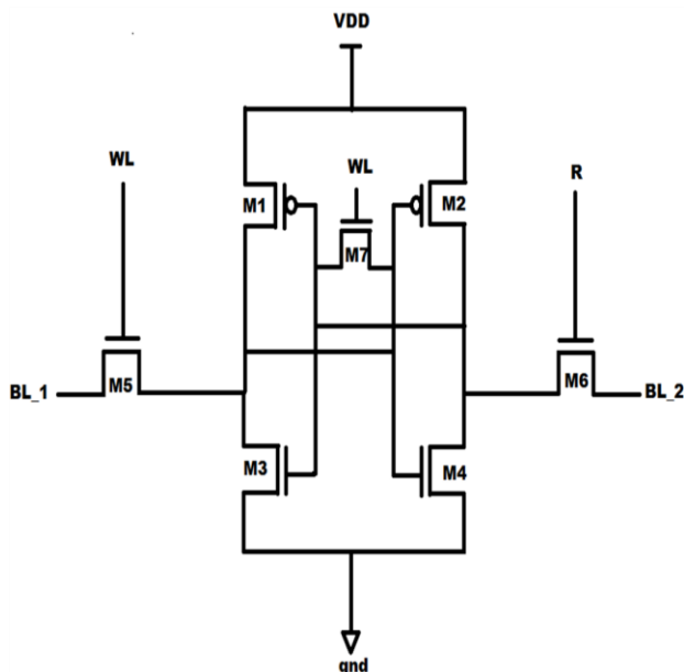
Fig. 2. 7T SRAM
