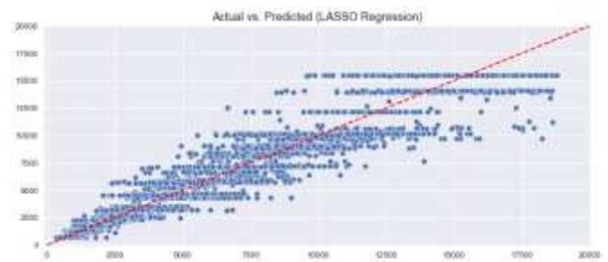
Fig. 17. Actual vs. Predicted
