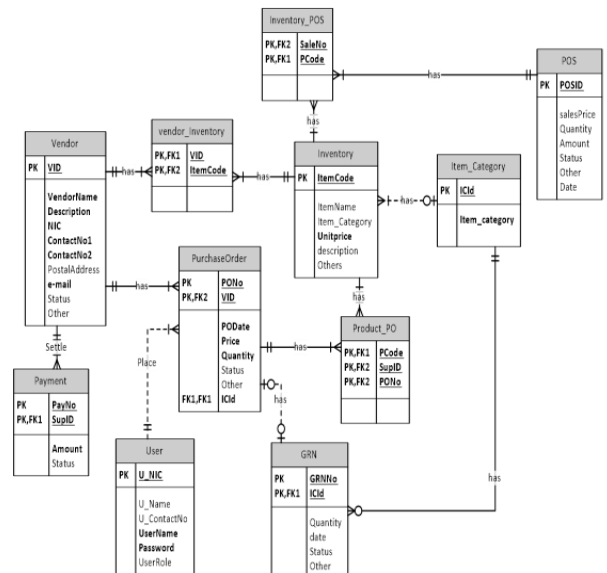
Figure 3. ER diagram
