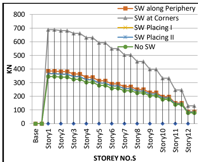
Fig.17. Storey Shear
