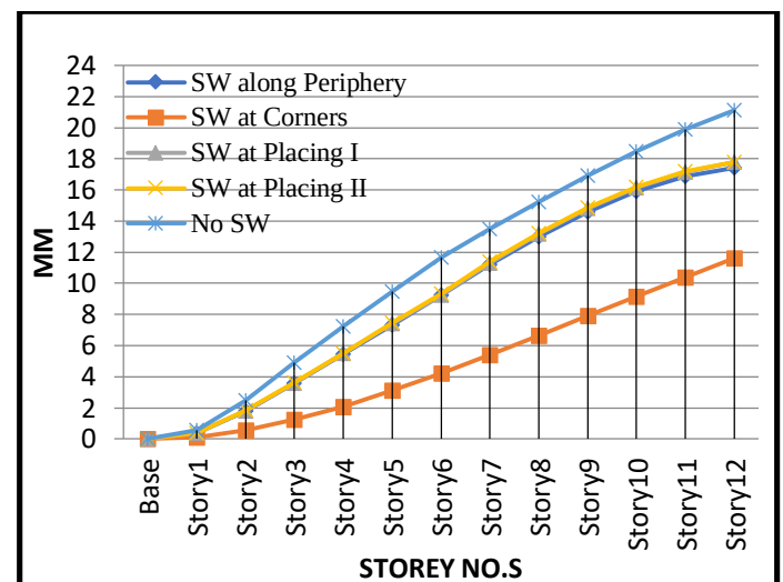
Fig.12. Storey Displacement
