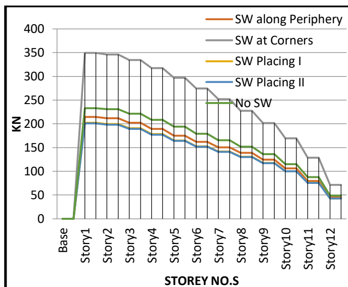
Fig.18. Storey Shear
