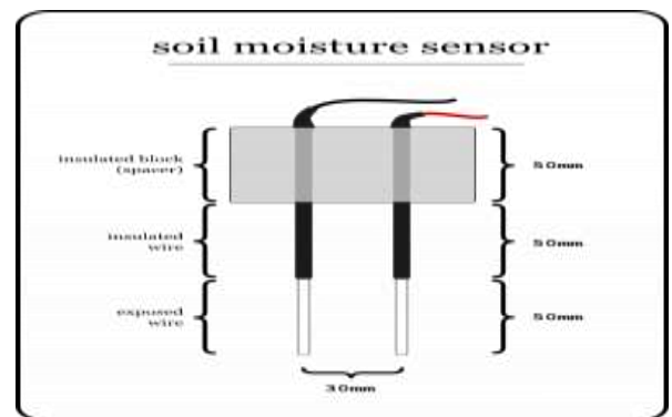
Fig.3. Moisture sensor
