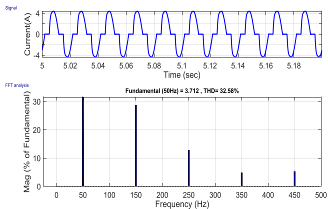
Fig. 10. (d) Current THD ( THD_i ) of fan
